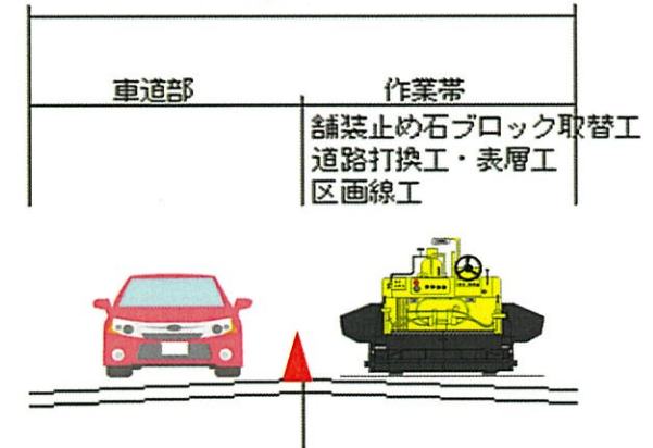
標準横断図
